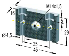
UM14 *€ 17,89 Universalfansch
