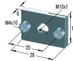
RF10 *€ 13,58 Rechteckflansch
