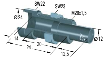
BV20 *€ 50,50 Bolzenvorlagerung
