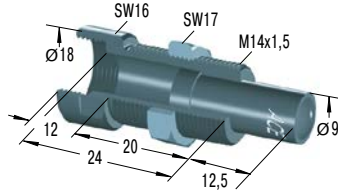
BV14 *€ 44,10 Bolzenvorlagerung
