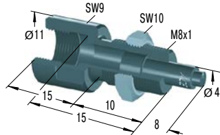
BV8 *€ 31,58 Bolzenvorlagerung
