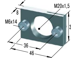
RF20 *€ 17,62 Rechteckflansch
