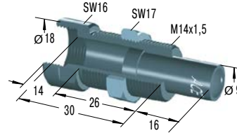
BV14SC *€ 45,56 Bolzenvorlagerung
