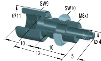
BV8A *€ 31,58 Bolzenvorlagerung
