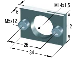
RF14 *€ 16,96 Rechteckflansch
