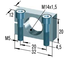
MB14 *€ 16,96 Klemmflansch
