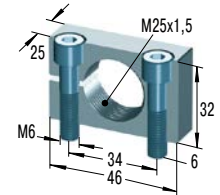
MB25 *€ 25,04 Klemmflansch
