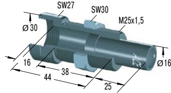
BV25 *€ 56,50 Bolzenvorlagerung
