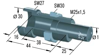
BV25SC *€ 57,80 Bolzenvorlagerung
