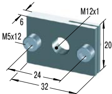
RF12 *€ 14,23 Rechteckflansch
