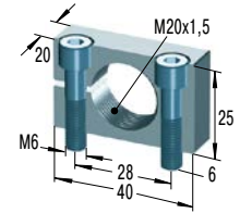
MB20 *€ 17,62 Klemmflansch
