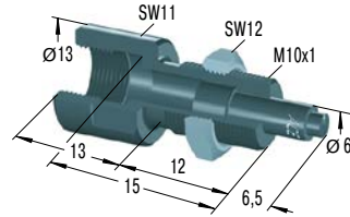
BV10 *€ 36,15 Bolzenvorlagerung
