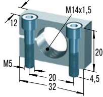
MB14 *€ 16,96 Klemmflansch
