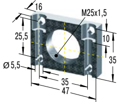
UM25 *€ 28,47 Universalfansch
