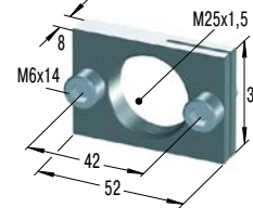
RF25 *€ 25,04 Rechteckflansch
