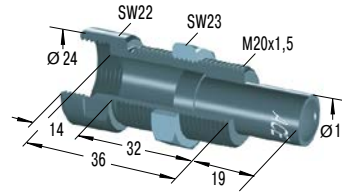
BV20SC *€ 52,59 Bolzenvorlagerung
