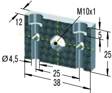
UM10 *€ 14,23 Universalfansch
