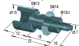
BV12SC *€ 38,24 Bolzenvorlagerung
